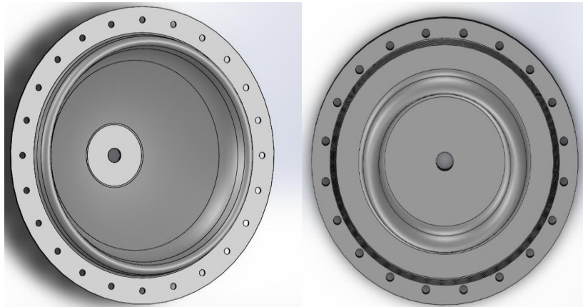
Şekil 5. Diyafram
