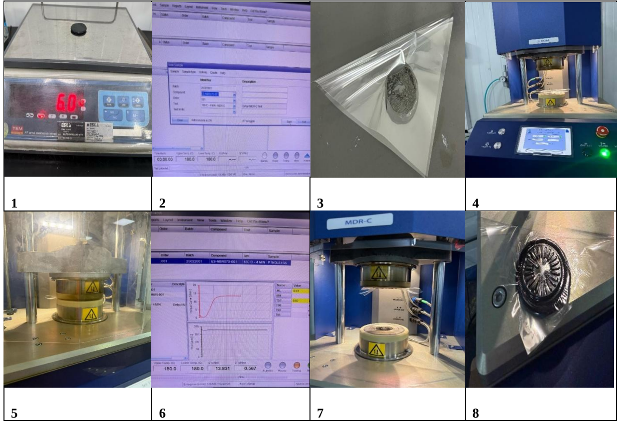
Şekil 3. Rheometer Ölçüm Hazırlık Aşamaları
