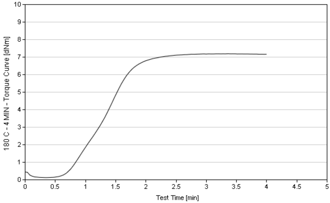
Şekil 2. Rheometer Pişme Grafiği
